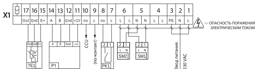
Схема внешних подключений
