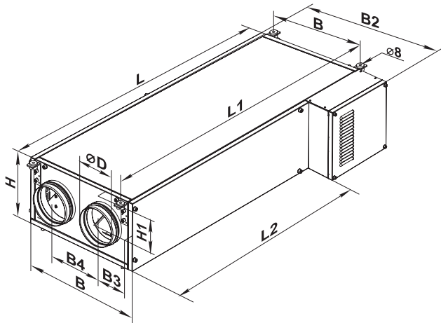
Рис.1 Габаритные размеры установки ВУТ 350 ПЭ ЕС
