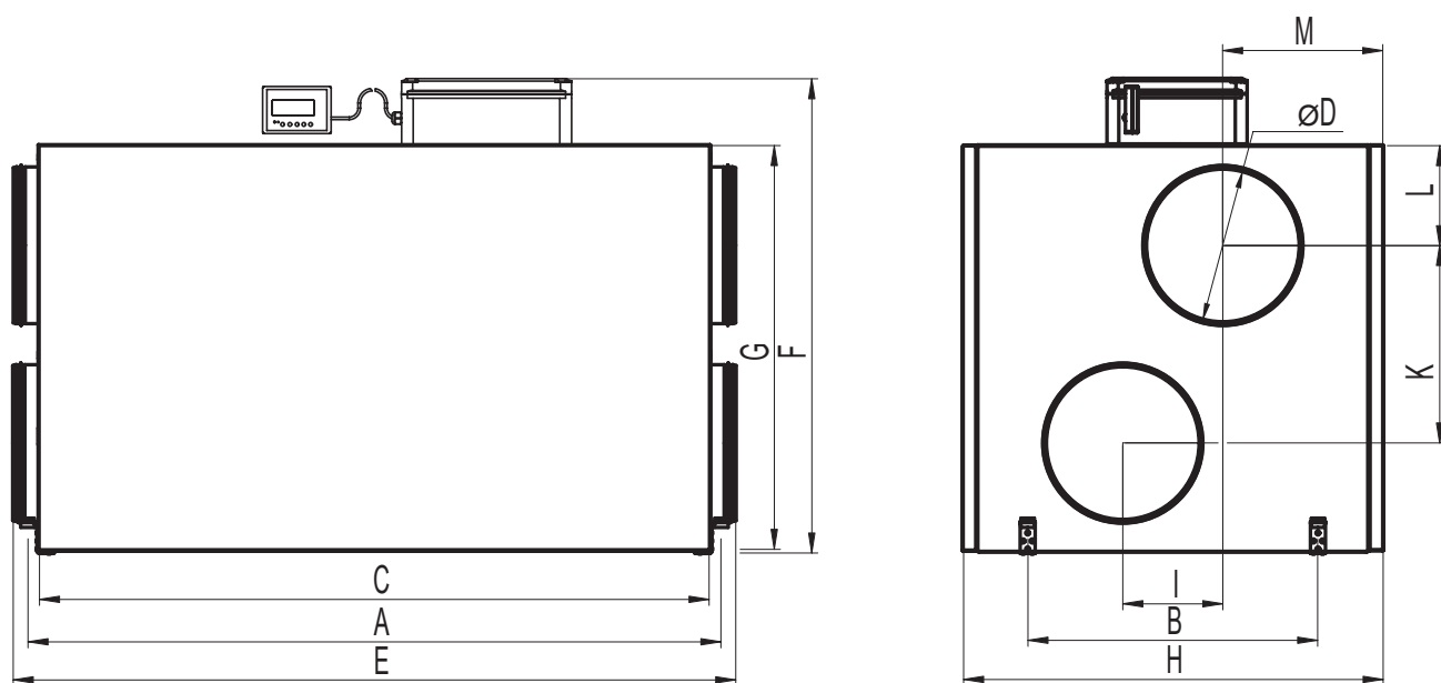
Рис. 2. Габаритные и присоединительные размеры для ВУТ ЭГ 800..2000
