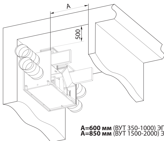
Рис. 6. Минимальные расстояния при монтаже установки
