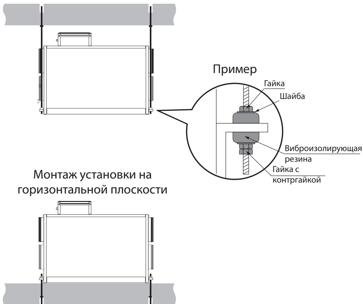
Рис. 5. Монтаж установки
