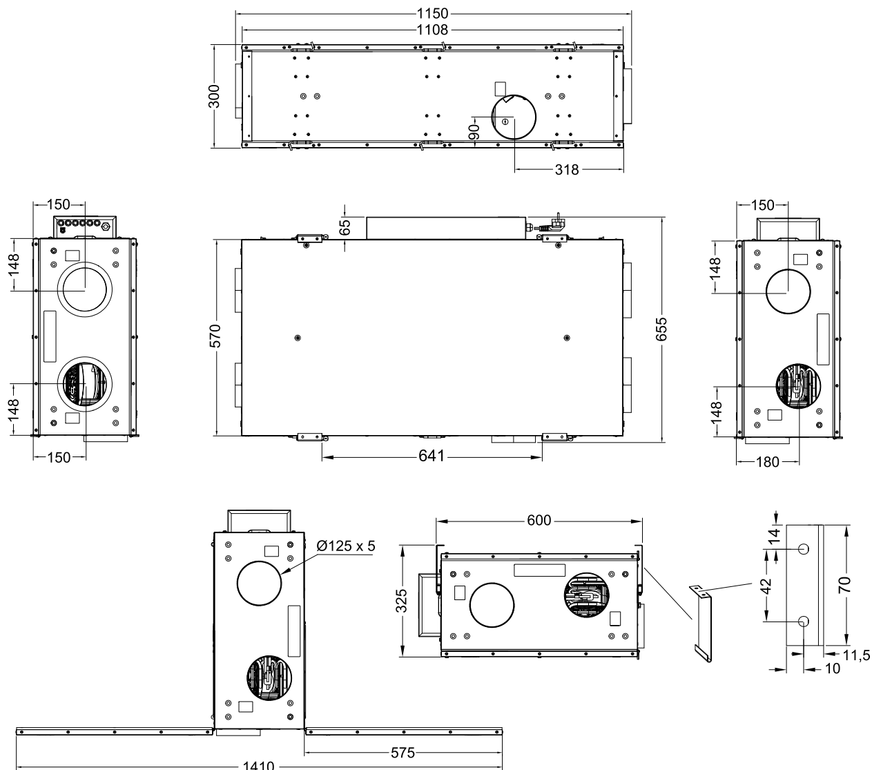
Рис. 1 Размеры
