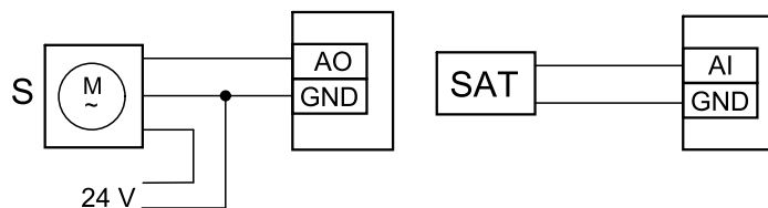
Рис. 16 Соединения канального охладителя
