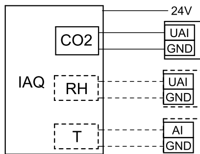
Рис. 13 IAQ соединения
