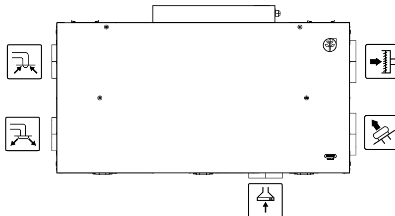
Рис. 2 Соединения воздуховодов
