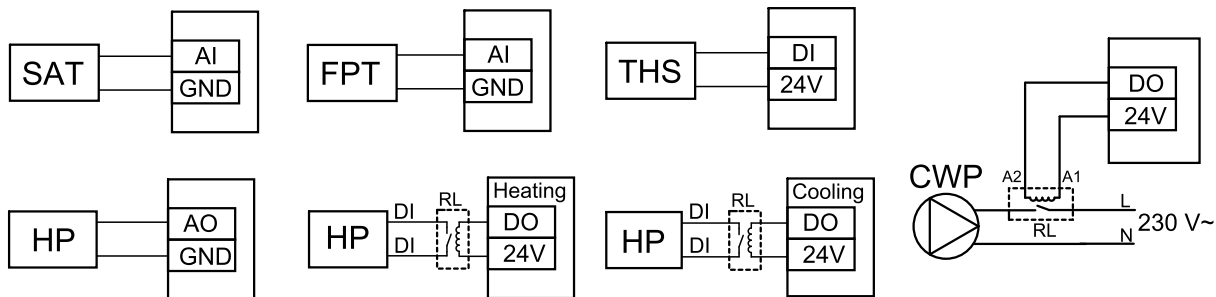
Рис. 17 Подключения переменного теплообменника холод/тепло
