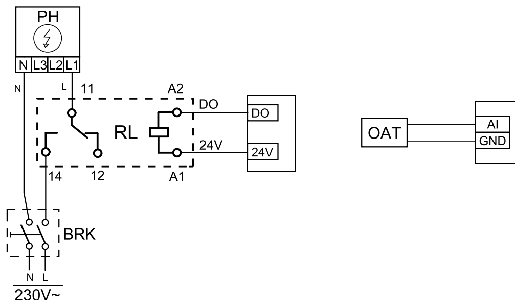
Рис. 14 Соединения предварительного нагревателя
