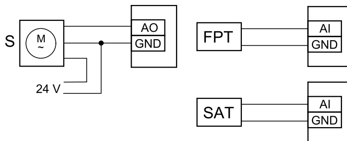
Рис. 15 Соединения водонагревателя
