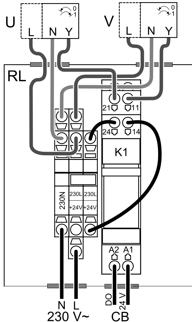
Рис. 18 Подключение клапана
