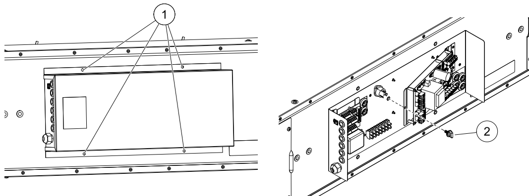
Рис. 4 Печатная плата
