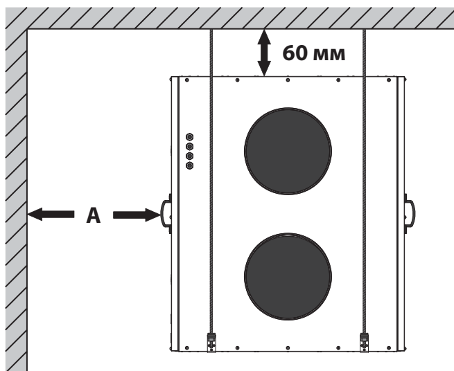
ПОДВЕСНОЙ МОНТАЖ
