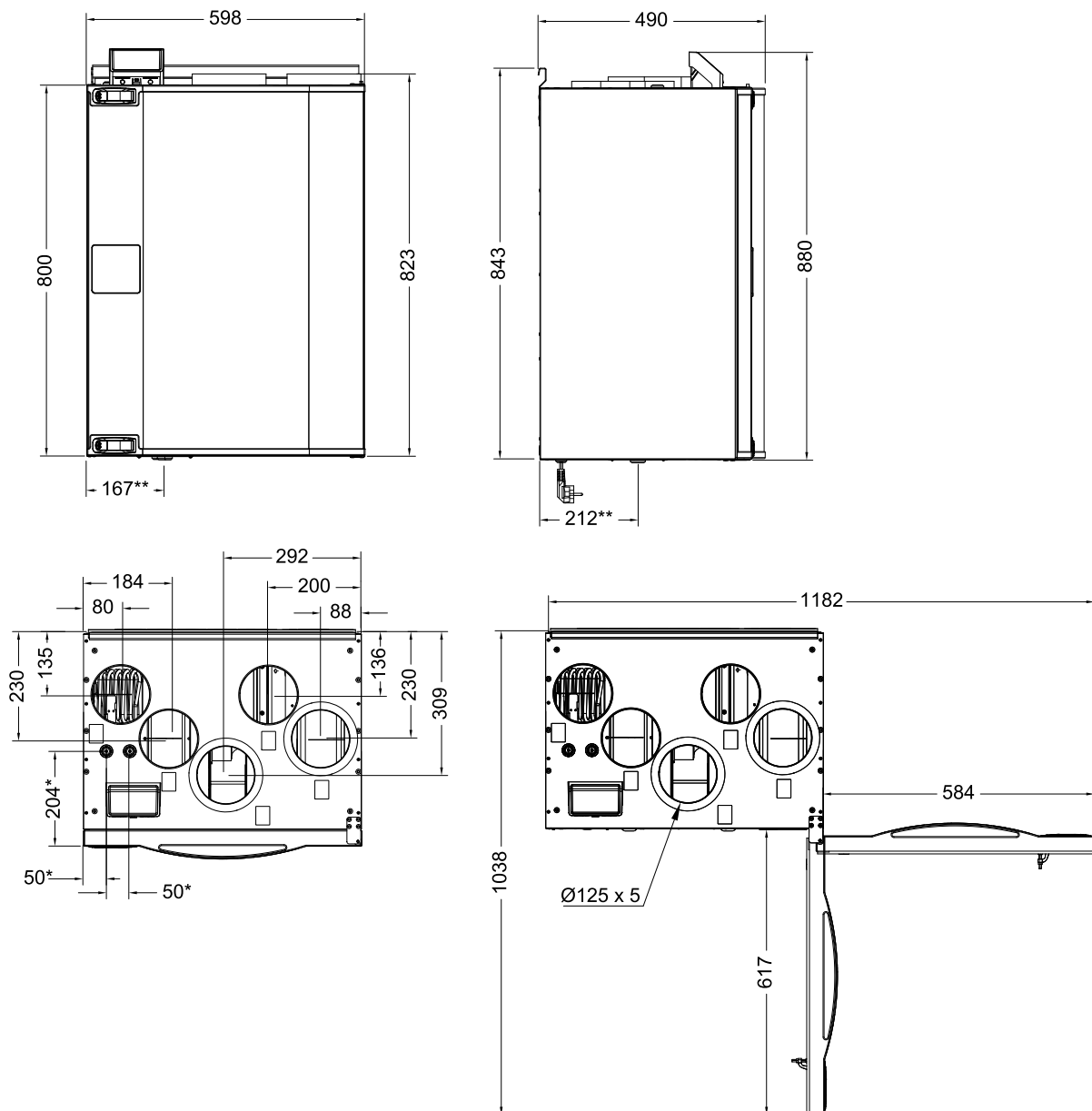
Рис. 1 Размеры левостороннего агрегата
