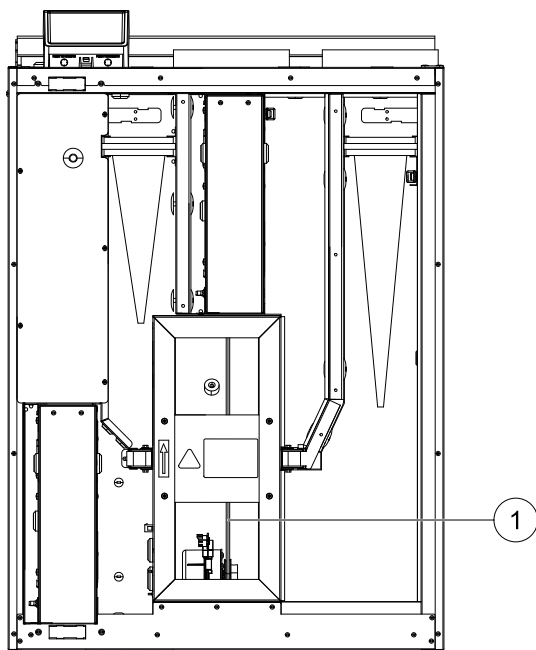
Рис. 11 Приводной ремень ротора
