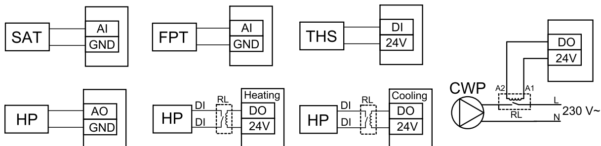
Рис. 18 Подключения переменного теплообменника холод/тепло
