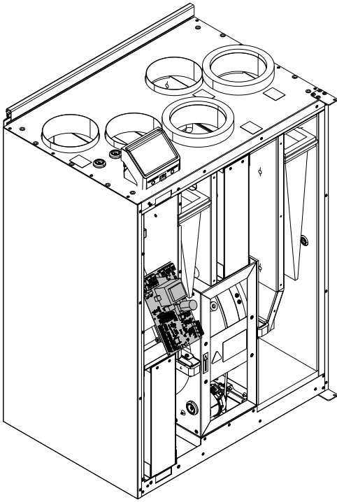
Рис. 6 Местоположение печатной платы
