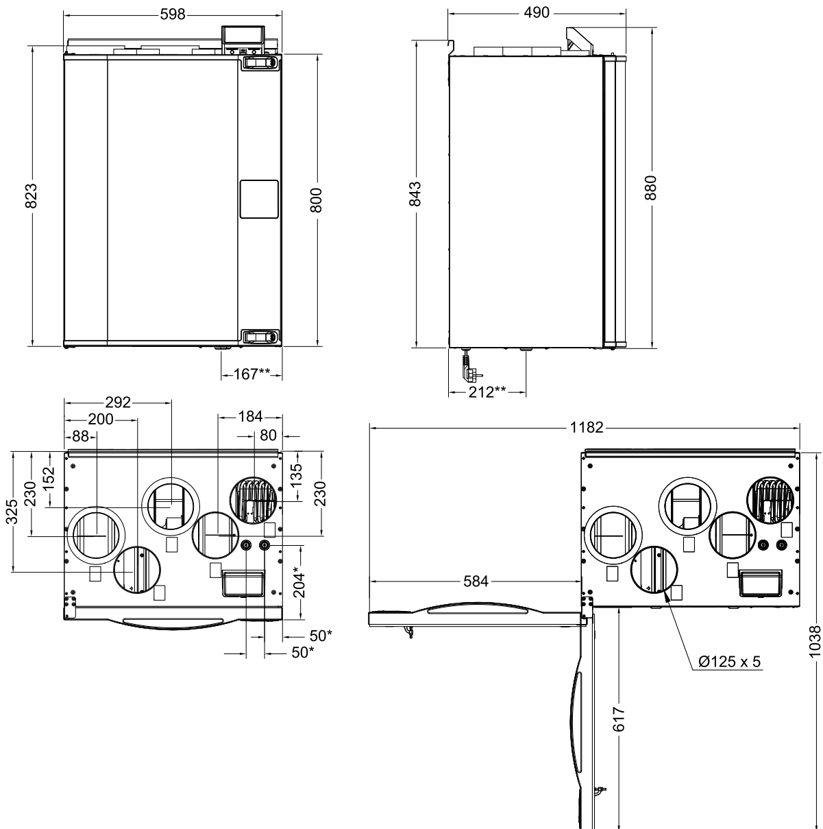
Рис. 2 Размеры правостороннего агрегата
