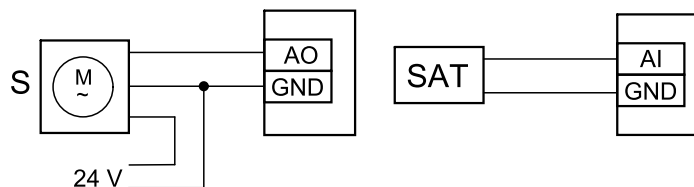
Рис. 17 Соединения канального охладителя
