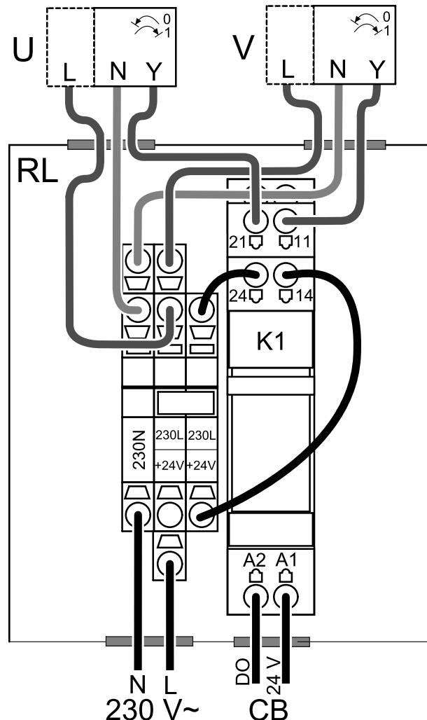
Рис. 19 Подключение клапана
