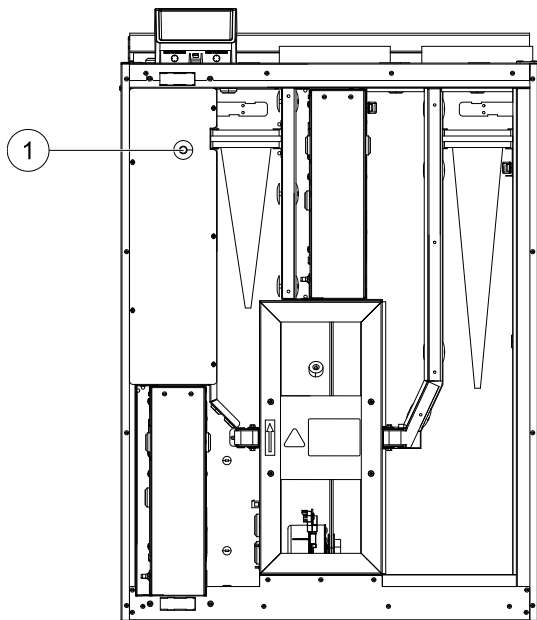
Рис. 10 Кнопка сброса защиты от перегрева
