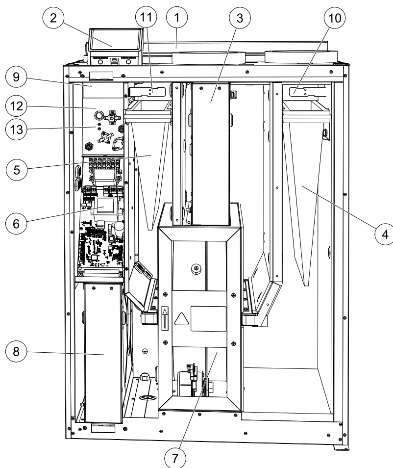
Рис. 9 Внутренние компоненты
